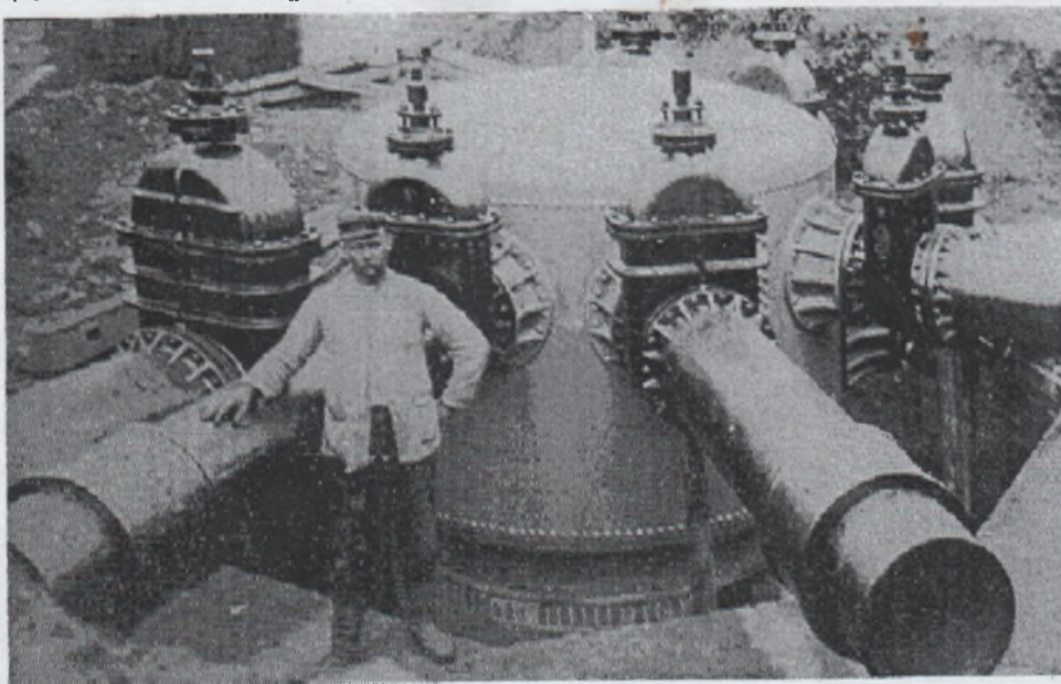
Via deze verdeelketel, die in 1902 wordt geplaatst onder het Nassauplein, komt het water uit de duinen naar Amsterdam. (foto Gem. Waterleidingbedrijf)
